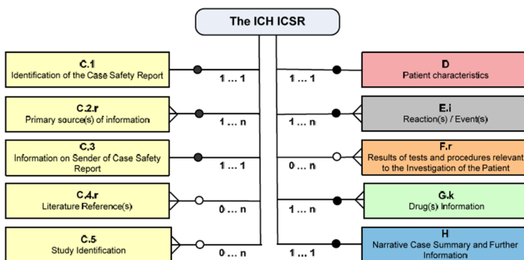
Figure 1. ICH ICSR data structure
